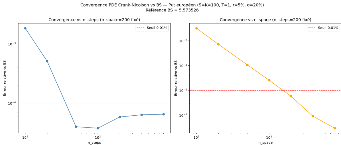
FIGURE 29 – Convergence PDE Crank-Nicolson vs BS — erreur relative en fonction de n_{\text{steps}} (gauche, n_{\text{space}} = 200 fixé) et de n_{\text{space}} (droite, n_{\text{steps}} = 200 fixé). La ligne rouge matérialise le seuil 0,01%.
