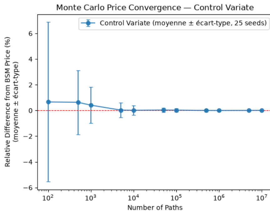
FIGURE 25 – Convergence - Variable de contrôle. Réduction de variance d'un facteur 2,6\times ; les barres d'erreur sont plus étroites que pour les variables antithétiques à paramètre égal.
