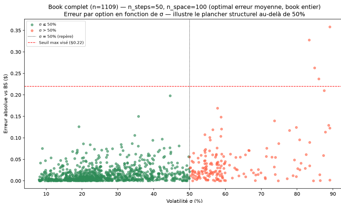
FIGURE 31 – Erreur absolue par option en fonction de la volatilité \sigma , aux paramètres optimaux ( n_{\text{steps}} = 50 , n_{\text{space}} = 100 ). La séparation nette à \sigma = 50\% illustre empiriquement le plancher structurel : 929 options à \sigma \leq 50\% (vert, erreur moy. $0,015, max $0,198) vs 180 options à \sigma > 50\% (orange, erreur moy. $0,043, max $0,358).
