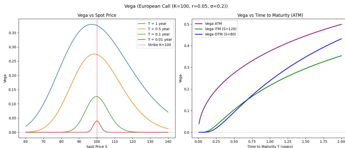
FIGURE 20 – Sensibilité du Vega - Call Européen
