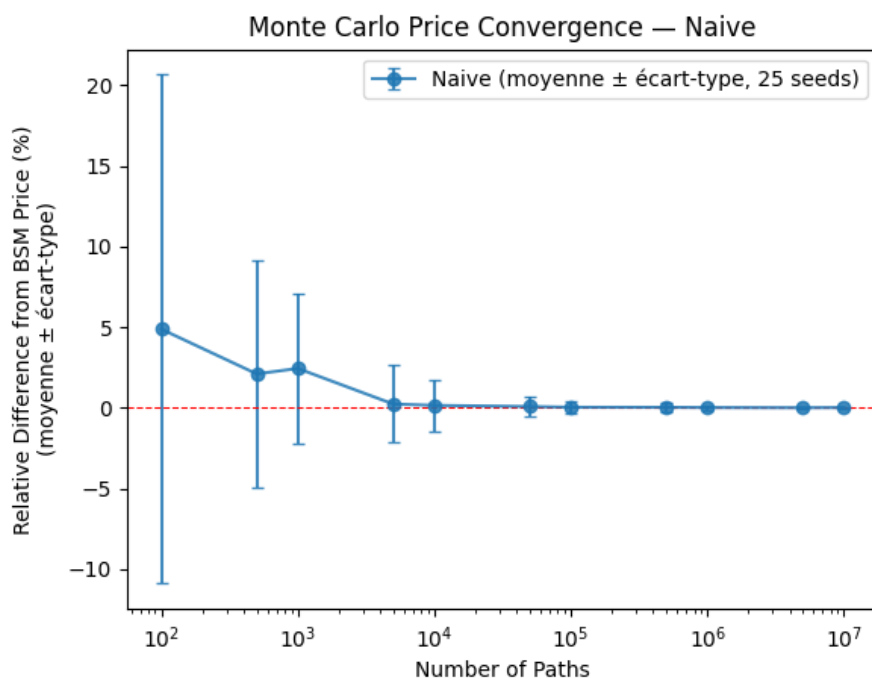
FIGURE 23 – Convergence de l'erreur relative (biais moyen \pm dispersion d'un tirage unique) - Monte Carlo naïf. La dispersion décroît en O(1/\sqrt{n}) , conformément au théorème central limite.
