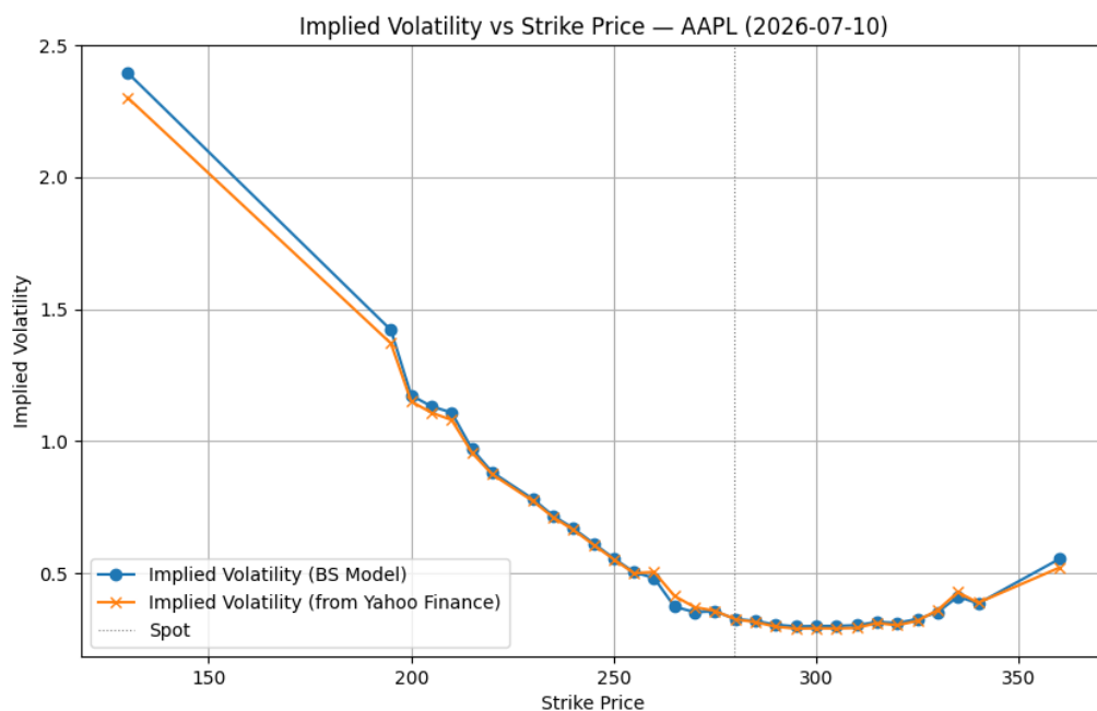
FIGURE 34 – Volatilité implicite calculée à partir du prix milieu ( mid-price ), sur options avec cotation active - comparaison avec la valeur fournie par Yahoo Finance
