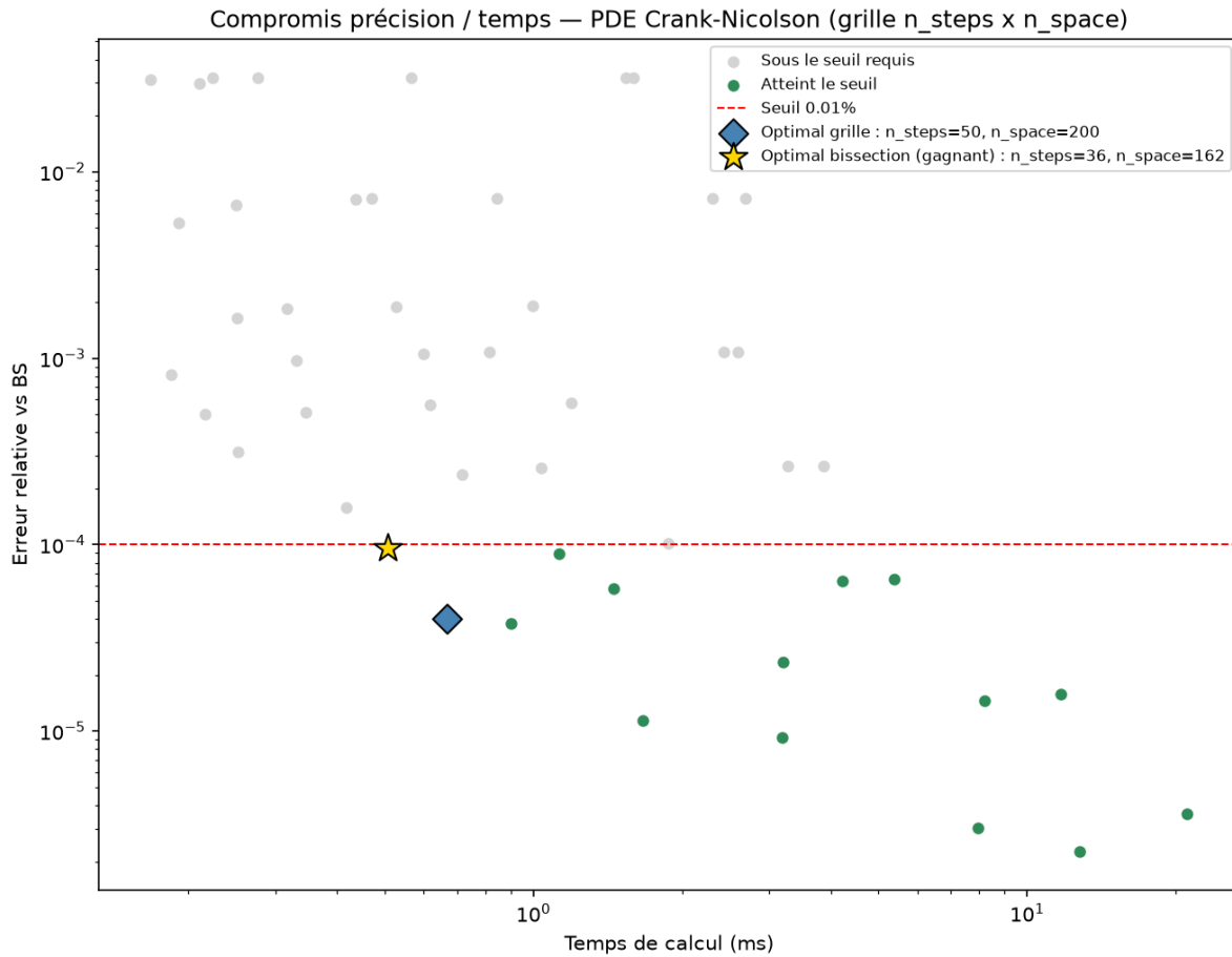
FIGURE 30 – Compromis précision/temps sur cas unique — configurations atteignant le seuil 0,01% (vert), optimal balayage (losange bleu) et optimal bisection (étoile jaune).
