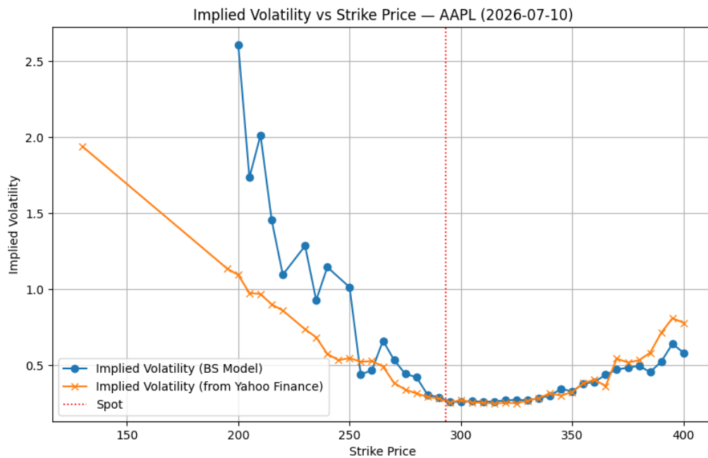
FIGURE 33 – Volatilité implicite calculée à partir du dernier prix traité ( lastPrice ) — forte divergence pour les strikes ITM lointains
