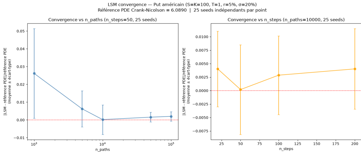
FIGURE 27 – Convergence LSM : erreur relative moyenne \pm écart-type sur 25 seeds, vs n_{\text{paths}} (gauche) et vs n_{\text{steps}} (droite)
