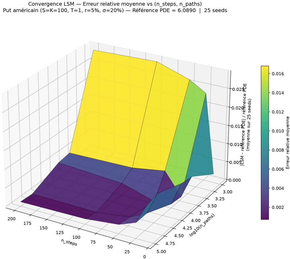
FIGURE 28 — Surface d'erreur relative moyenne (25 seeds) en fonction de (n_{\text{steps}}, \log_{10}(n_{\text{paths}})) , Put américain ( S = K = 100 , T = 1 , r = 5\% , \sigma = 20\% ), référence PDE = 6,0890
