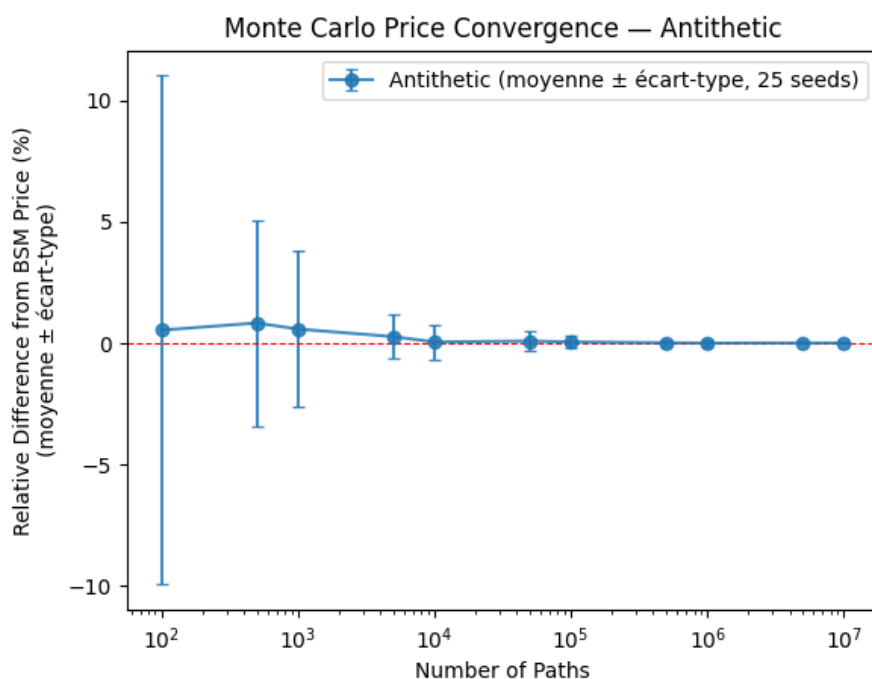
FIGURE 24 – Convergence - Variables antithétiques. La réduction de dispersion d'un facteur 2\times par rapport au naïf (à n fixé) est clairement visible : les barres d'erreur sont deux fois plus étroites.
