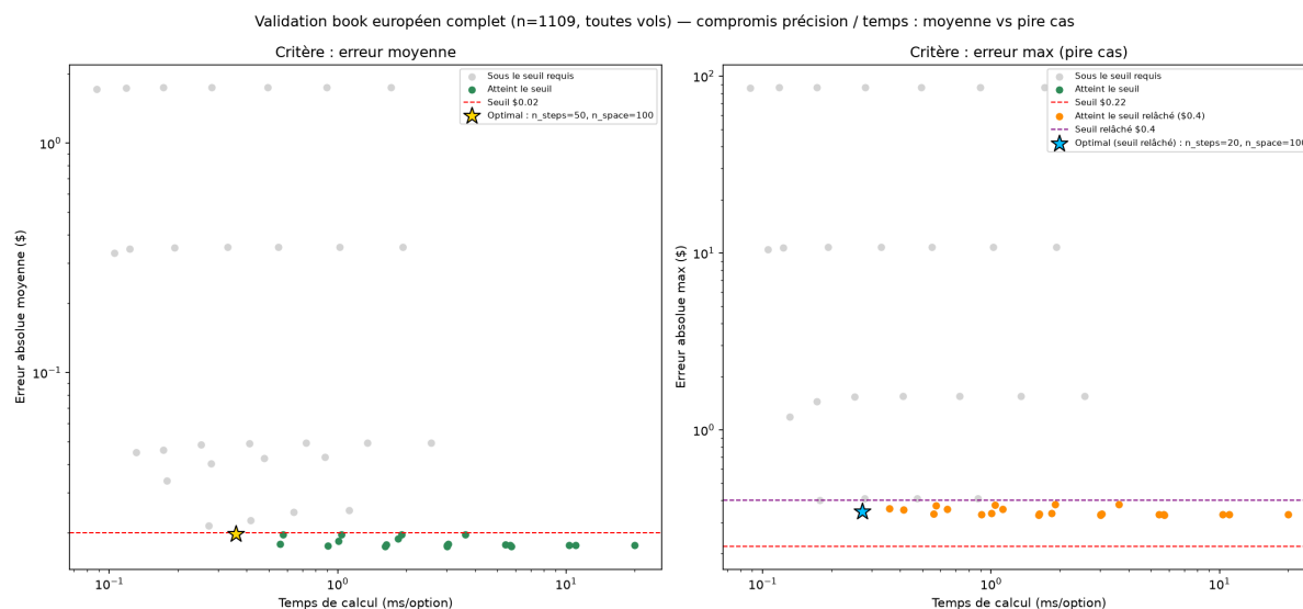
FIGURE 32 – Compromis précision/temps sur le book complet (1 109 options). Gauche : critère erreur moyenne, optimal à n_{\text{steps}} = 50 , n_{\text{space}} = 100 (étoile jaune). Droite : critère erreur maximale, aucune configuration ne passe le seuil strict $0,22 (rouge) ; l'optimal au seuil relâché $0,40 (violet) est à n_{\text{steps}} = 20 , n_{\text{space}} = 100 (étoile bleue).
